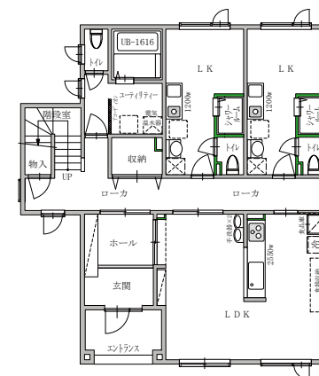
1 階平面図
