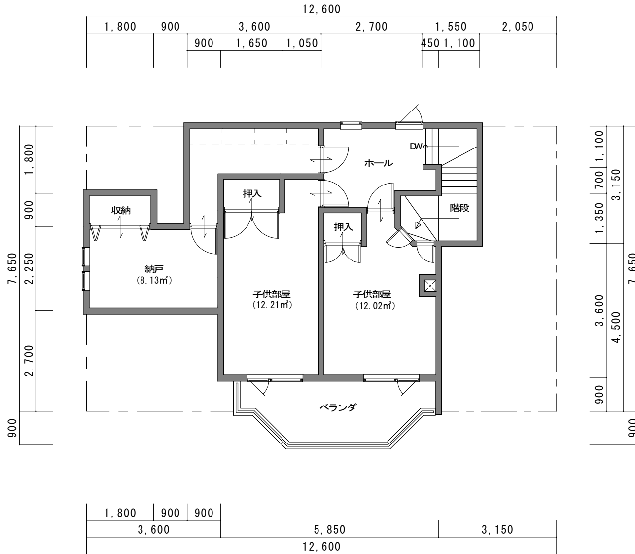
2階 1/100
