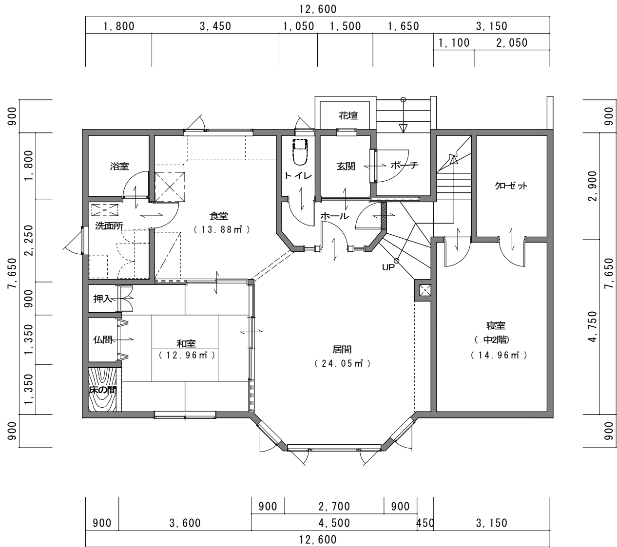
1階 1/100
